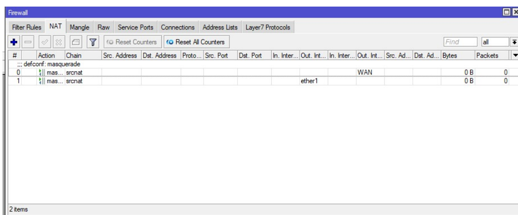
Gambar 11: konfigurasi NAT
